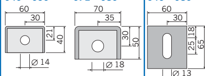
Deckenaufhänger ceiling hangers
