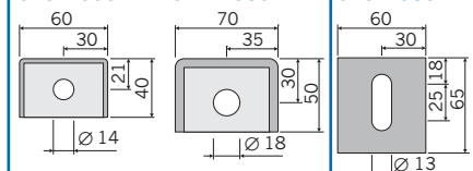
Baugröße / Size 040 - 050 071 - 080
